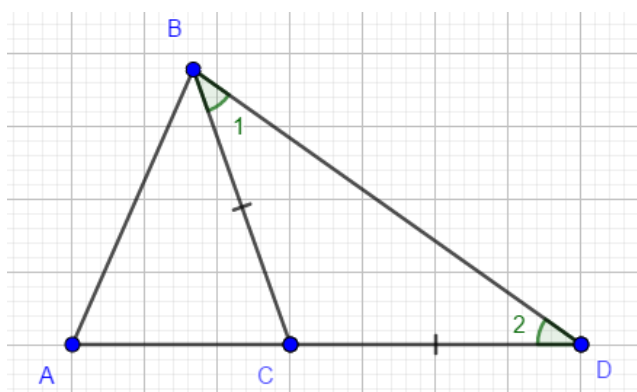
Рисунок 55 – Неравенство треугольника
