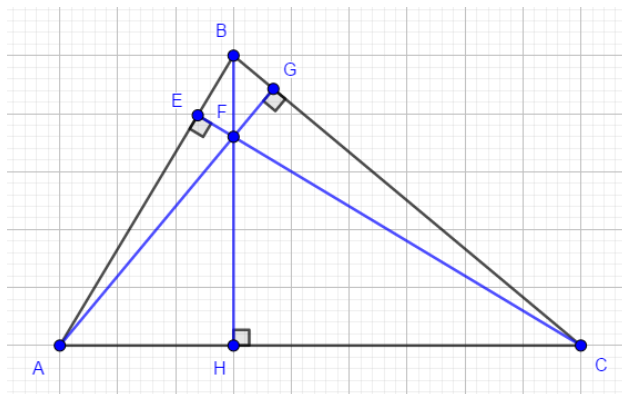
Рисунок 52 – Ортоцентр треугольника
