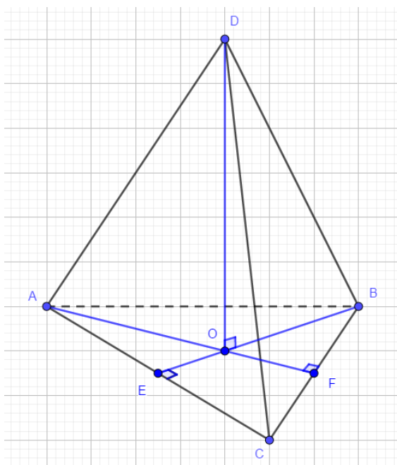
Рисунок 78 – Ортоцентрический тетраэдр
