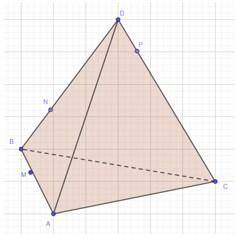
Рисунок 92 – Данный тетраэдр
