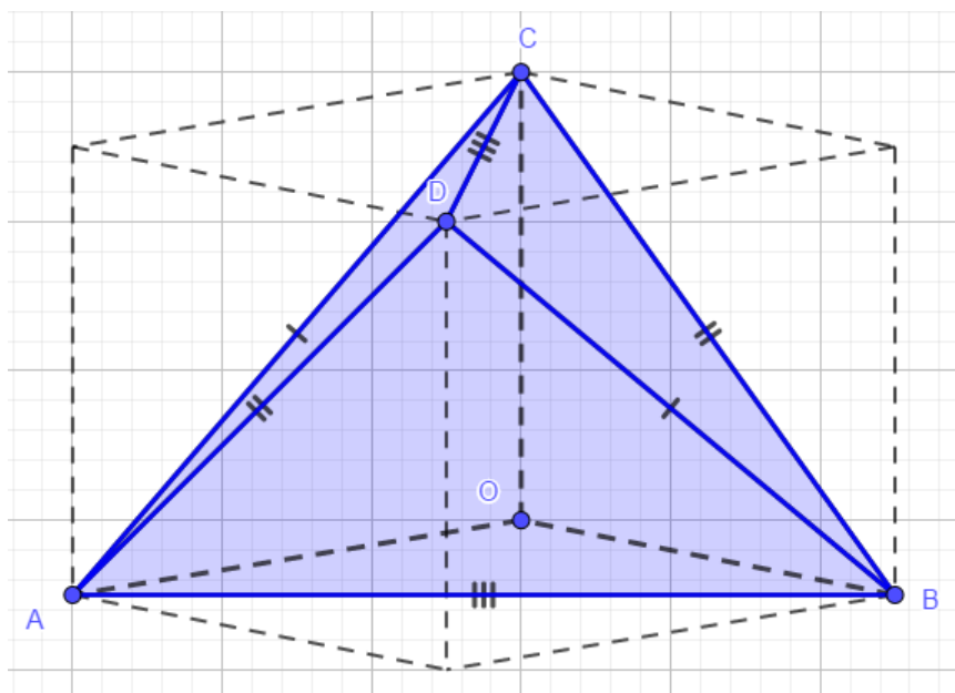
Рисунок 77 – Равногранный тетраэдр
