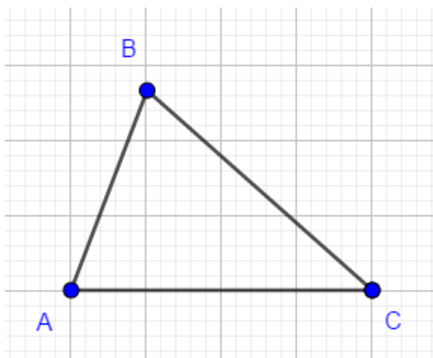
Рисунок 56 – Треугольник ABC
