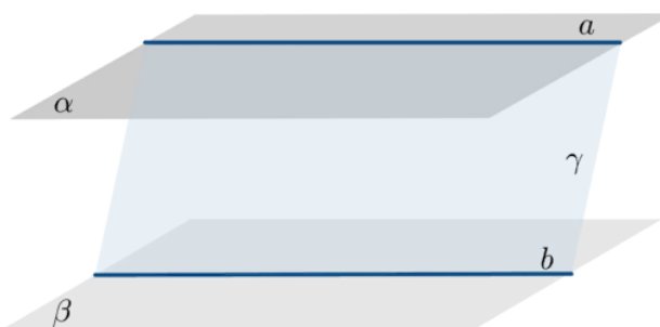
Рисунок 86 – Пересечение плоскостей
