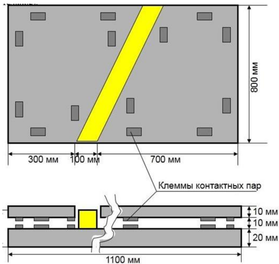
Рисунок 4 – Финишная площадка для учебной башни
