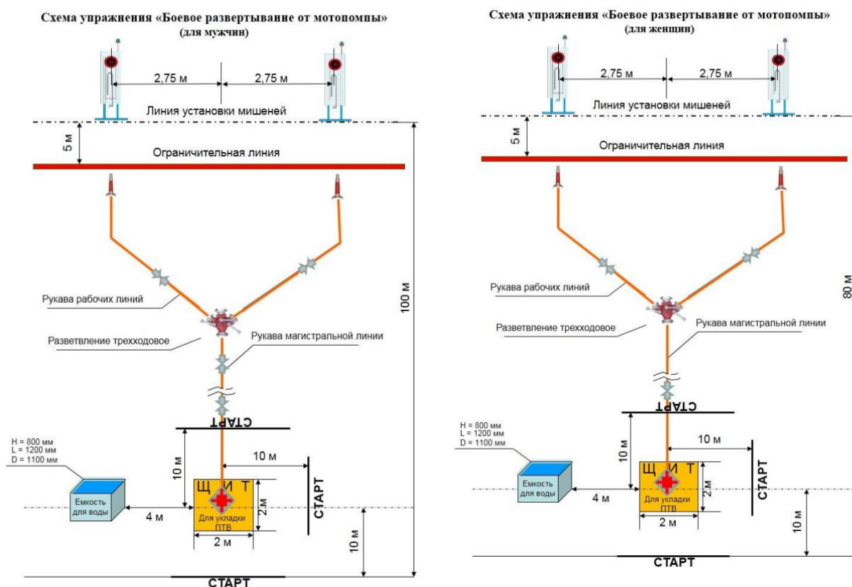
Рисунок 1 – Схема упражнения «Боевое разворачивание»
